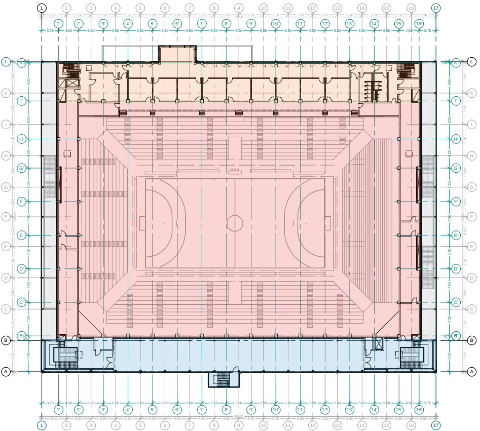
Grundriss 2. Obergeschoss
