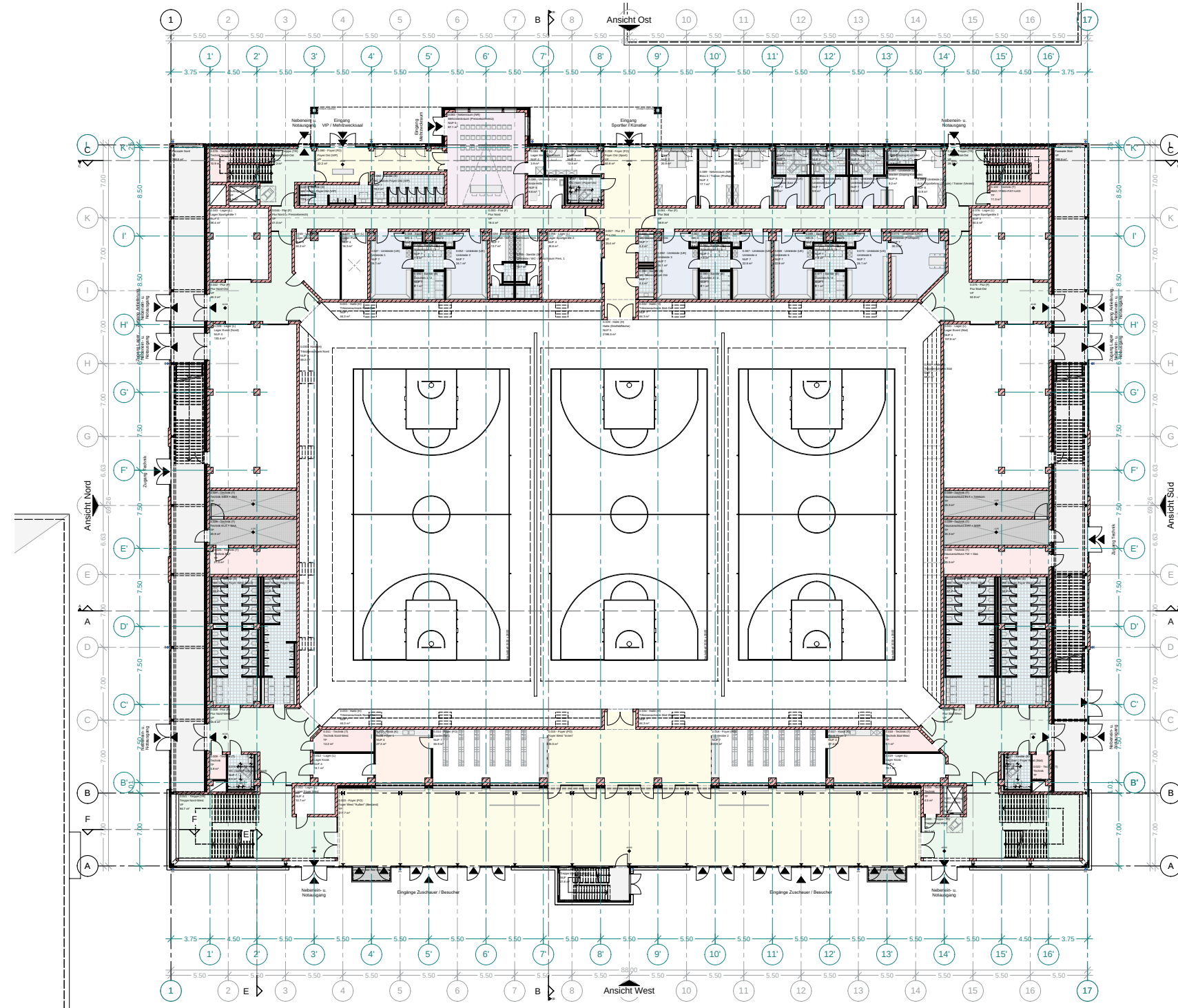
Grundriss Erdgeschoss (Übersicht)
