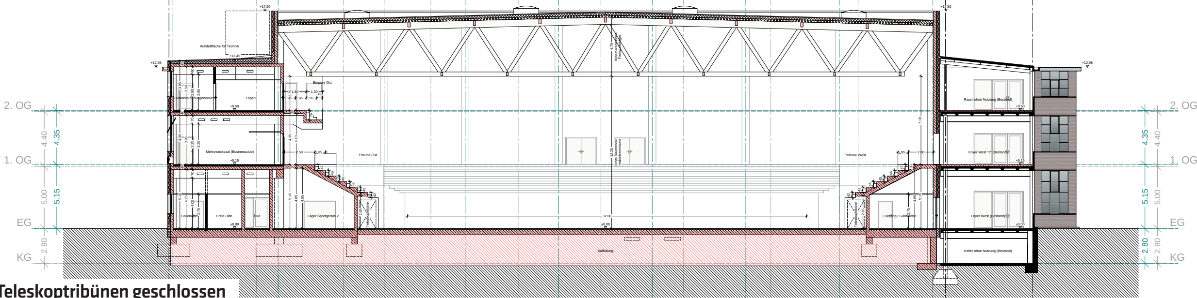
Schnitt B-B, Teleskoptribünen geöffnet
