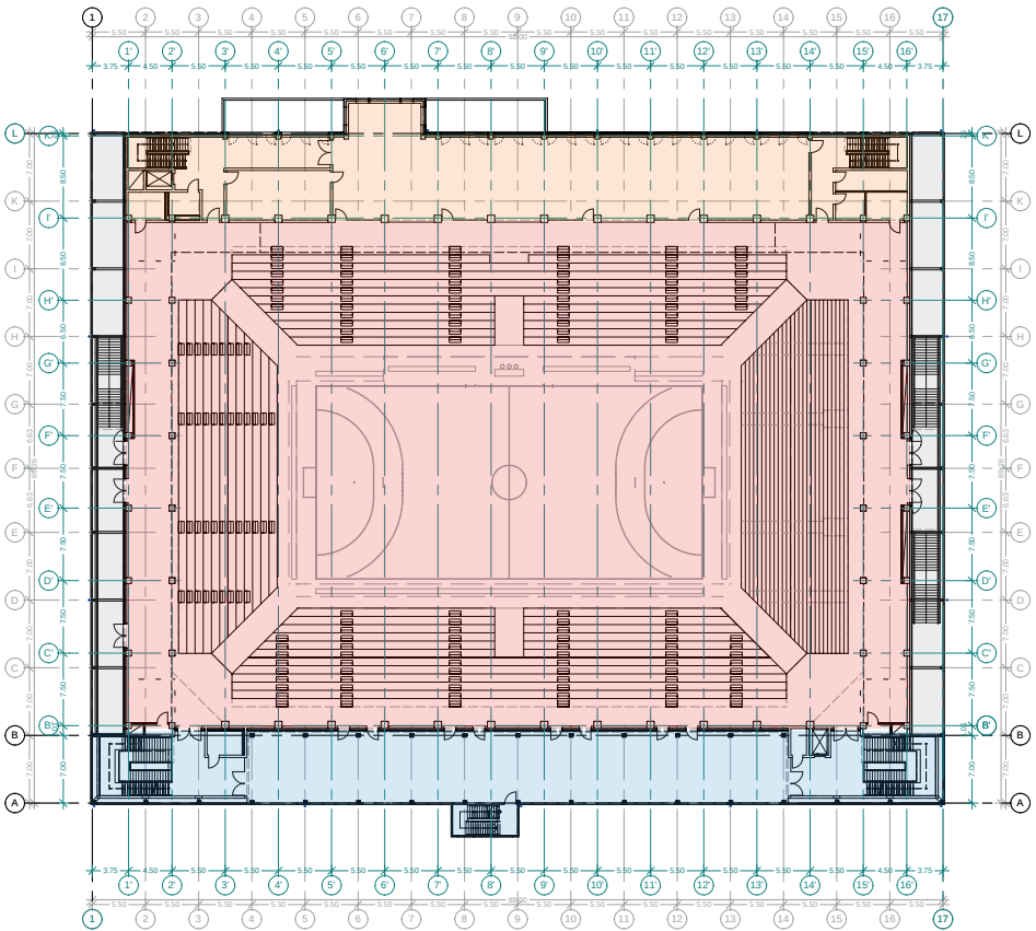
Grundriss 1. Obergeschoss
