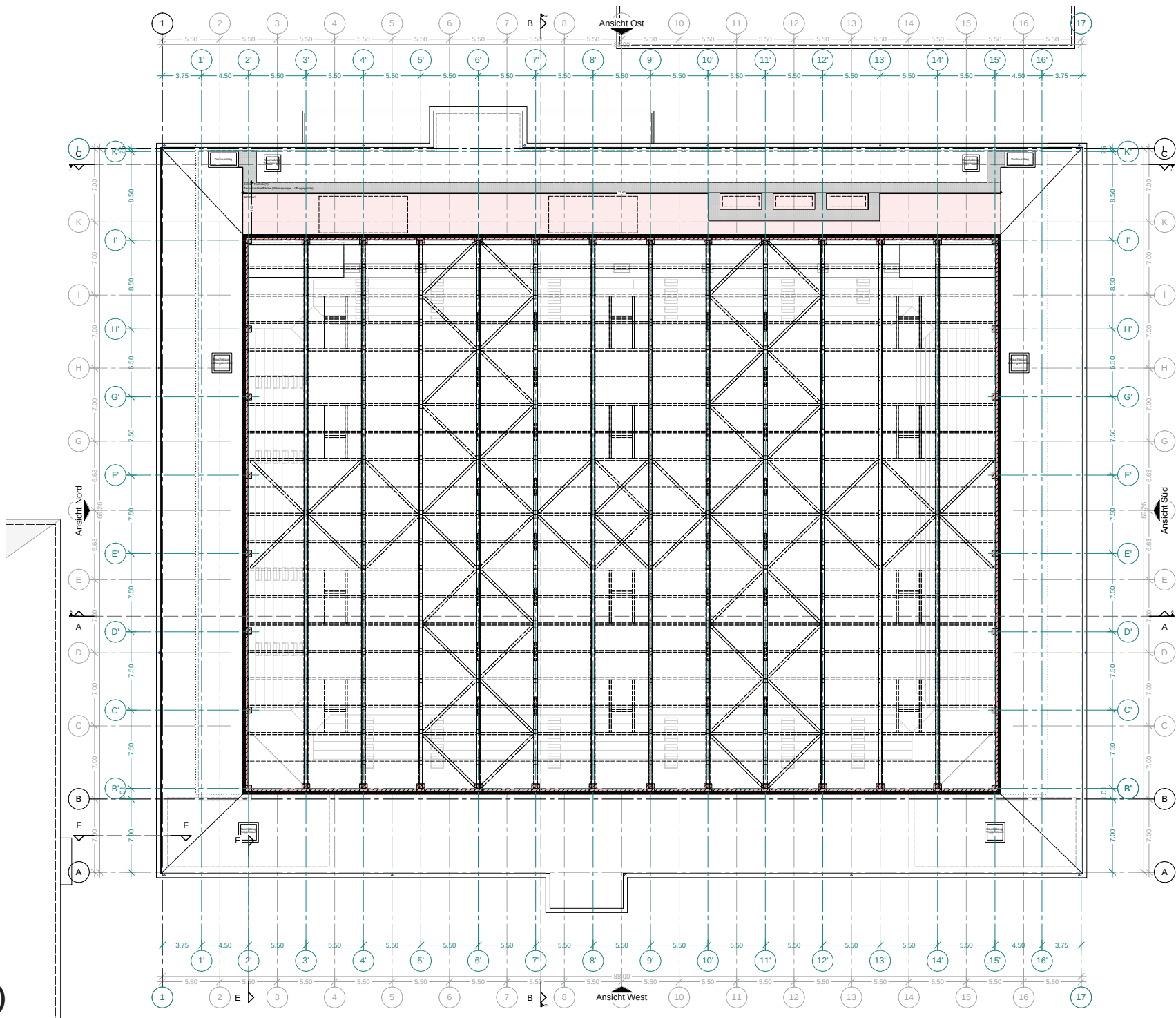
Grundriss Dachgeschoss (Übersicht)
