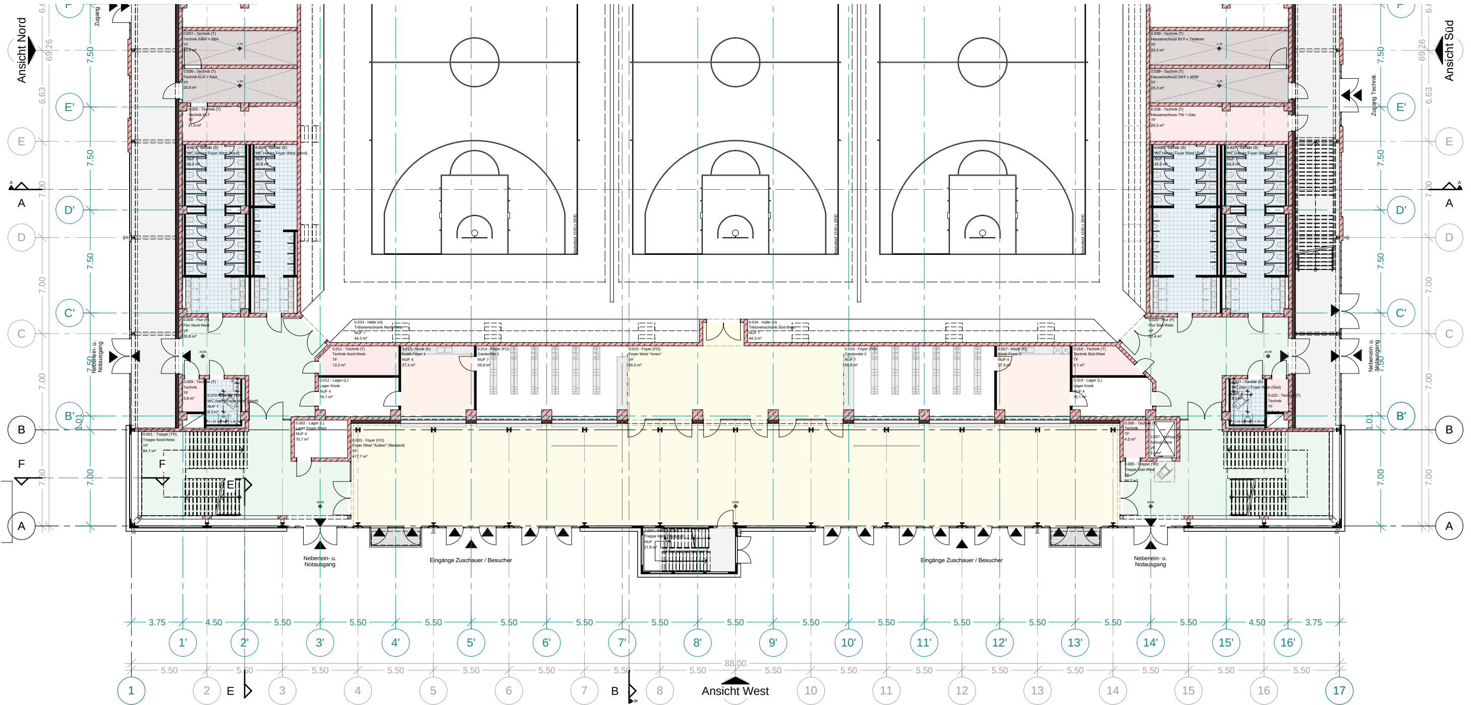
Grundriss Erdgeschoss (Ausschnitt West)
